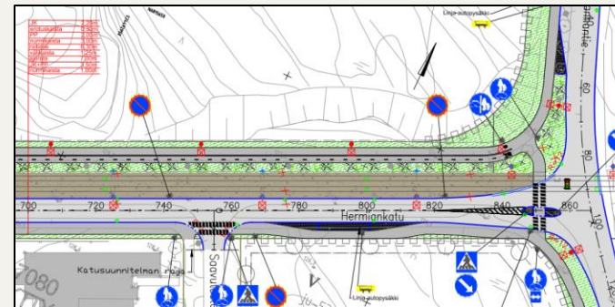
Kuva: Hermiankadun 2. raide.
