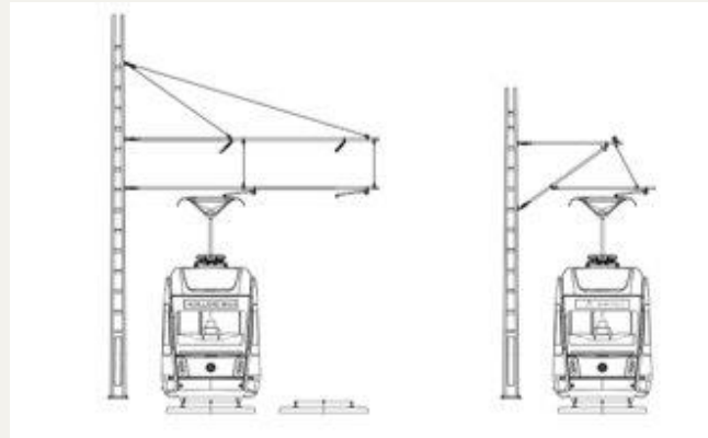
Kuva: Kääntöorsi
