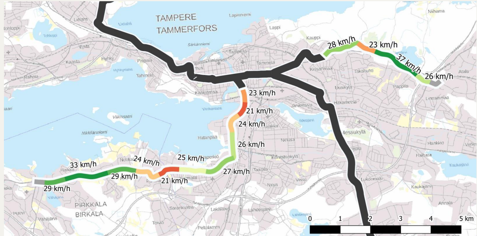
Kuva: Raitiotien keskinopeudet osuuksittain.
