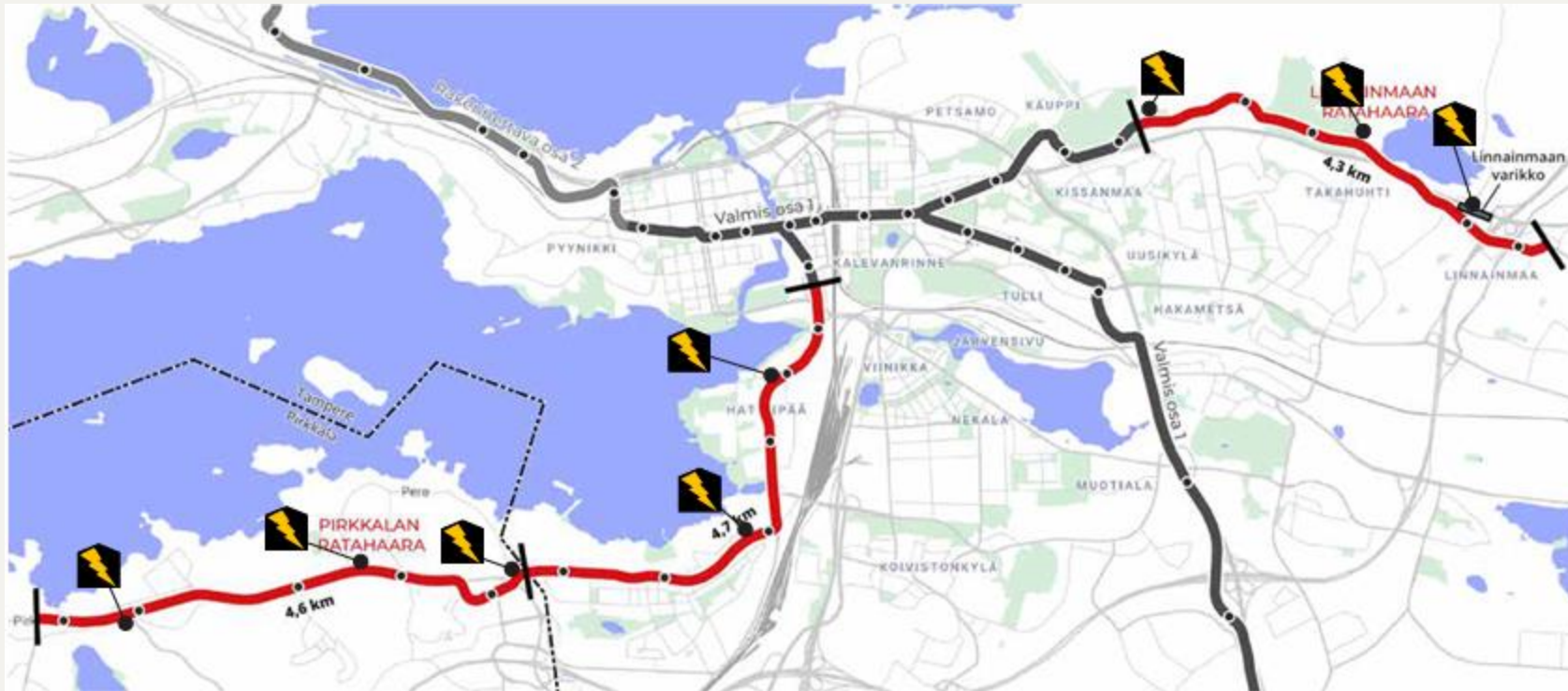
Kuva: Hankesuunnitelman sähkösyöttöasemien sijainnit.
